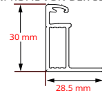
RAHMENPROFIL VON DER SEITE
