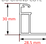
PROFIL DU GRAND CÔTÉ
