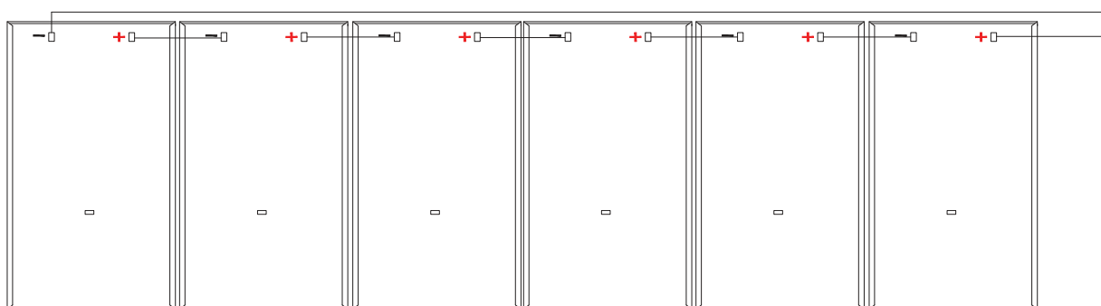
Leapfrog-Verkabelung (Hochformat)
