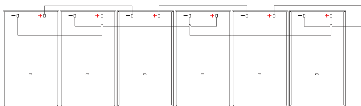
Querformatige Verkabelung
